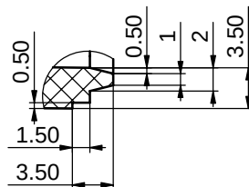
局部视图 C 比例 2.4:1
