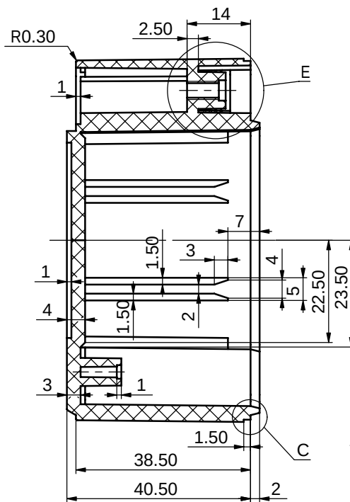
剖面 A-A
