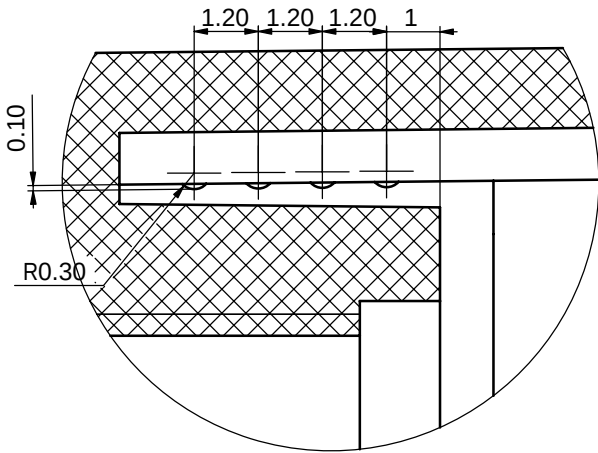
局部视图 F 比例 10:1
