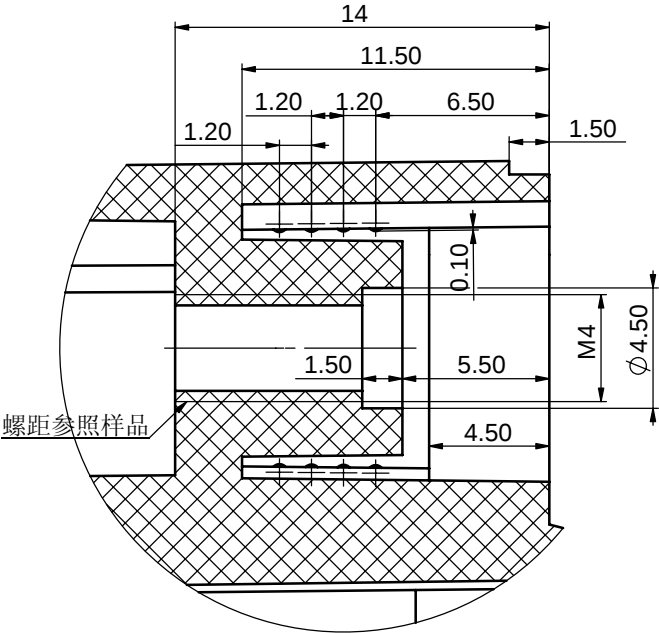
局部视图 E 比例 5:1
