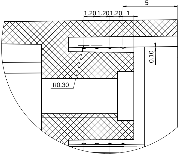
局部视图 F 比例 8:1
