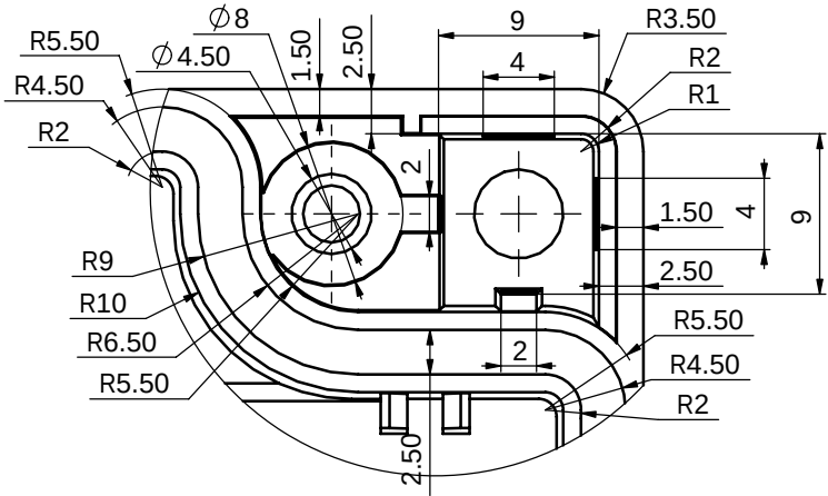
局部视图 C 比例 3:1
