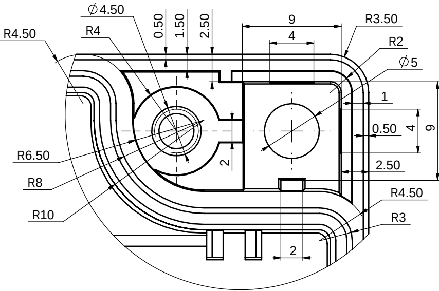
局部视图 D 比例 4:1
