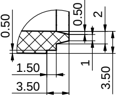
局部视图 C 比例 2.4:1
