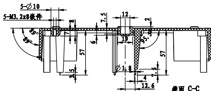
截面 C-C
