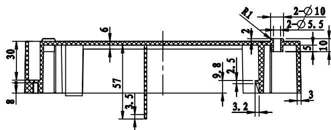
截面 B-B
