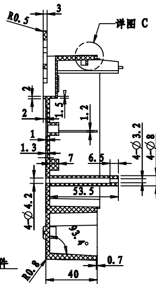
截面 A-A
