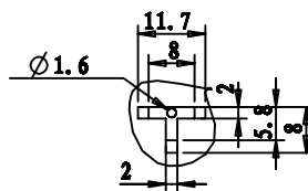
细节 D 刻度 1:1
