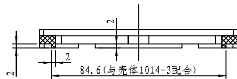
剖面 A-A
