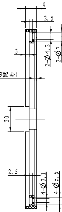
剖面 B-B
