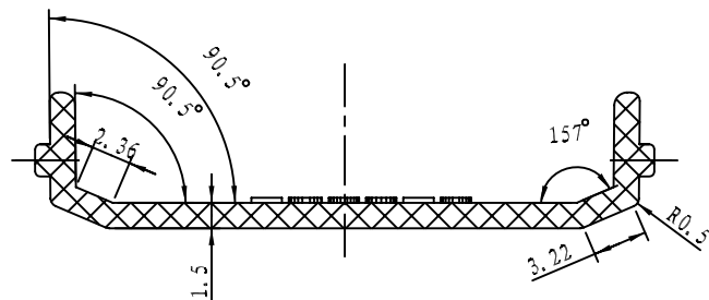
剖面 P-P
