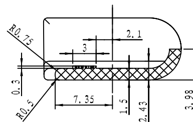
剖面 C-C
