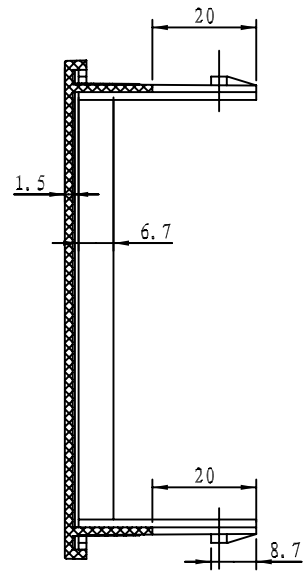
剖面 B-B
