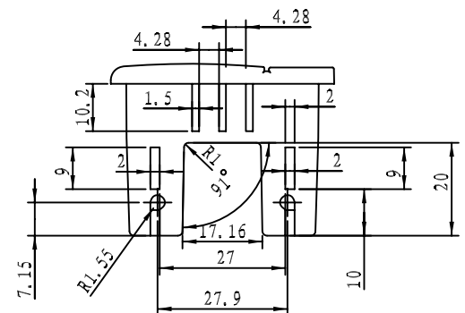
剖面 A-A
