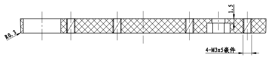
剖面 A-A
