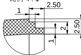
局部视图 B 比例 4:1
