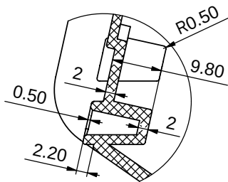
局部视图 C 比例 2:1.5
