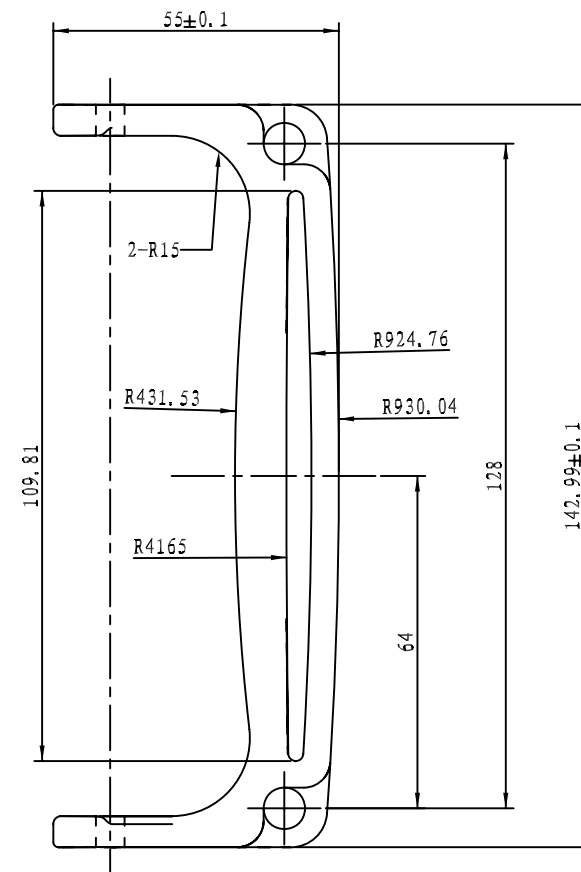
正面, 外表面
