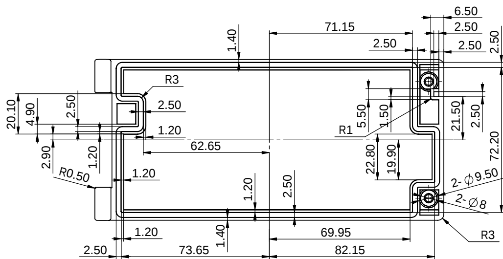
背面（顶杆面）
