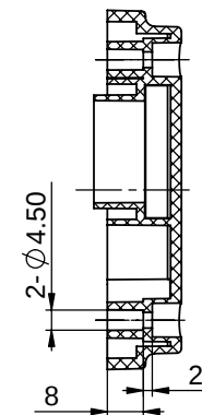
剖面 B-B
