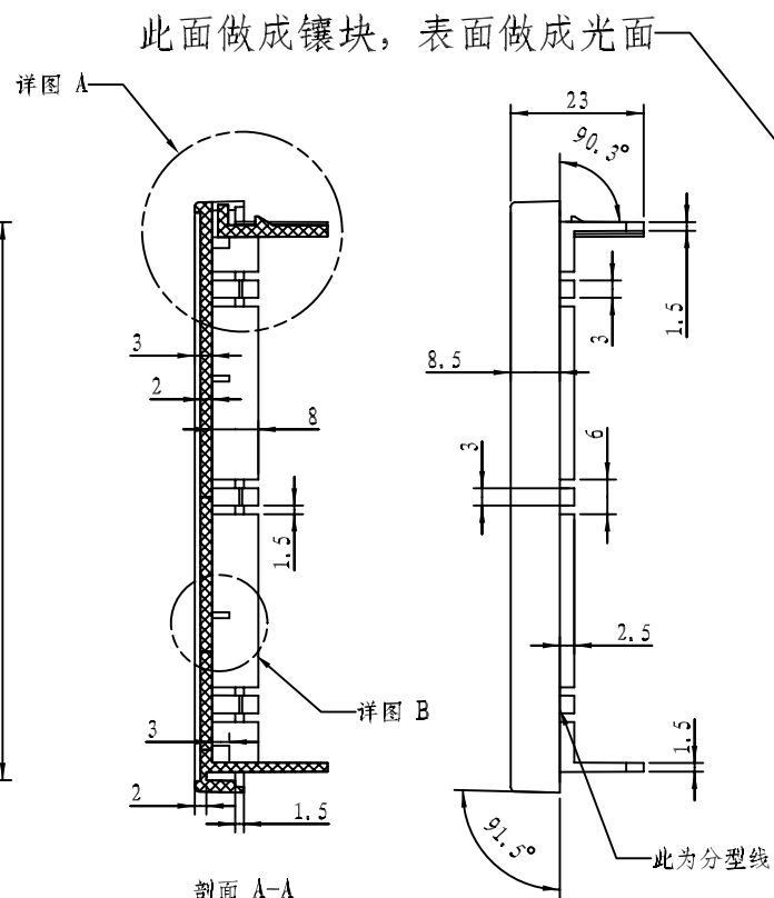
剖面 A-A
