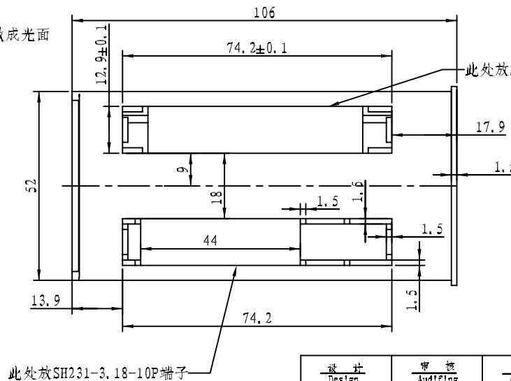
剖面 A-A
