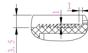
细节 A 比例 8:5
