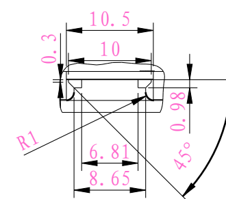
细节 B 比例 8:5
