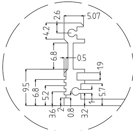
详细剖面A-A 比例2:1
