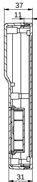
剖面 A-A
