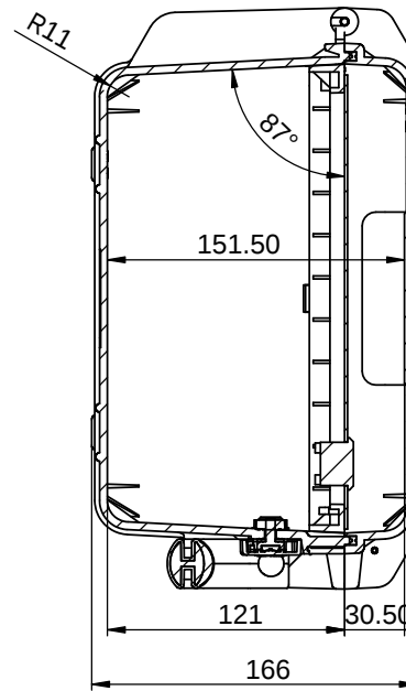
剖面 A-A
