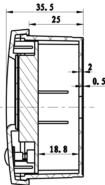
剖面 B-B
